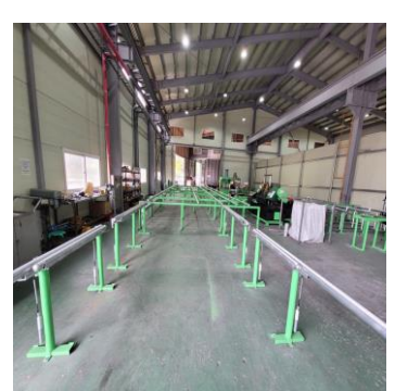
티뽑기 자동화라인
